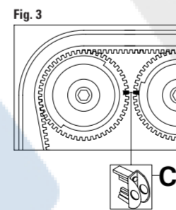
FIGURA 1 Verificar la correcta alineación de la marca de puesta a punto A. FIGURA 2 Verificar la correcta alineación de la marca de puesta a punto B. FIGURA 3 Insertar la herramienta especial de inmovilización de árbol de levas C.
