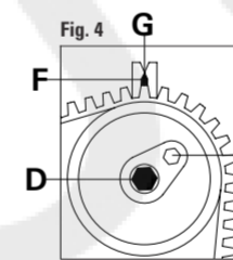
FIGURA 4 Aflojar el tornillo de fijación D. Girar el tensor de la correa sobre el excéntrico de regulación E, en sentido de las agujas del reloj hasta lograr que el indicador F quede alineado con la muesca de fase G. Por último, apretar el tornillo de fijación D. FIGURA 5 Aflojar el tornillo de fijación L. Girar el tensor de la correa sobre el excéntrico de regulación H en sentido de las agujas del reloj. Luego, alinear el indicador I con la muesca de fase M. Por último apretar el tornillo de fijación L.
