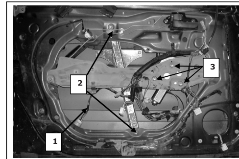
Porta lato destro, Portière avant droite, Right front door, Puerta lado derecho, Vorne rechte Tür, Porta frente dijeta, Sag on kapi, νότρα εμπρόσθια δεξιά
