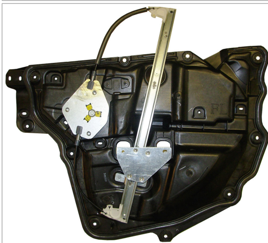
POWER WINDOW LEFT ALZACRISTALLI ELETTRICO SX A
