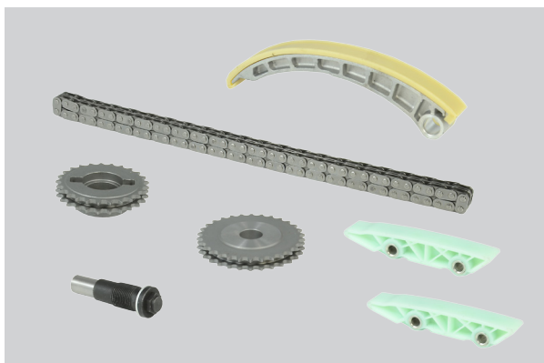
TCK195NG: Kette: Duplex, geschlossenes Glied, 84 Verknüpfungen
