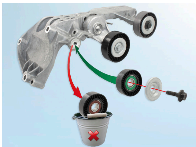
1. ábra: Feszítőegység 534 0243 10
