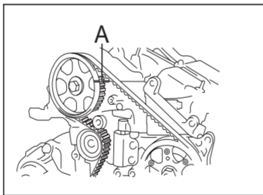
FIGURA 1 Extraer el tapón del cabezal de motor derecho A.
