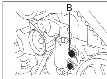
FIGURA 2 Aflojar los tornillos de fijación B del tensor de la correa, demónter las courroies de la distribución. FIGURA 3 Insertar la herramienta para inmovilización del tensor de correa C.
