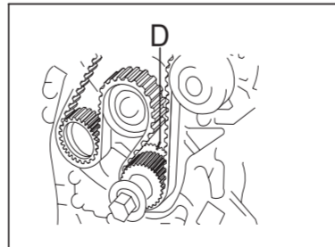
FIGURA 4: Verificar la correcta alineación de la marca de puesta a punto D.
