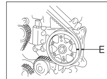
FIGURA 5: Verificar la correcta alineación de la marca de puesta a punto E.
