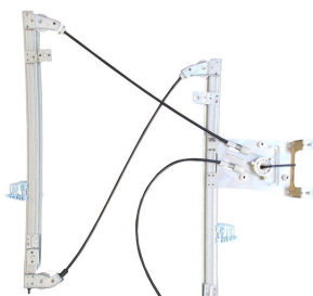
POWER WINDOW LEFT ALZACRISTALLI ELETTRICO SX
