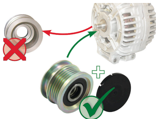
1. ábra: Váltás a merev szíjtárcsáról a generátor-szabadonfutóra
