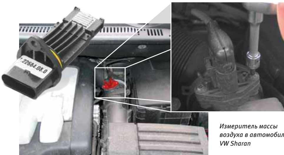
Вставка T 20 (6-лучевая, Torx®) с торцовым отверстием
