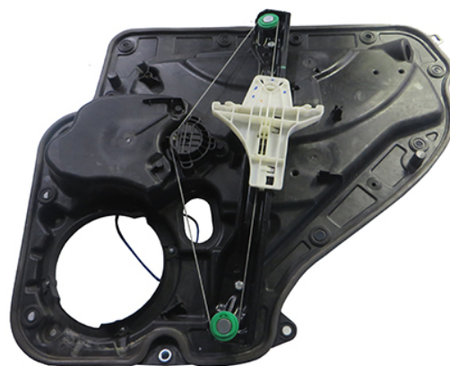
ORIGINAL POWER WINDOW ALZACRISTALLI ELETTRICO ORIGINALE
