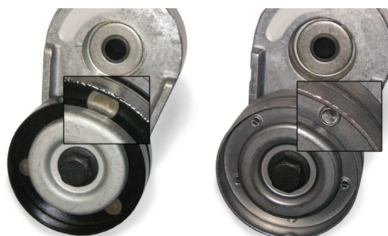
1. ábra: A futógörgők eddigi kivitelének (bal) és az új kivitelek (jobb) részletes nézete
