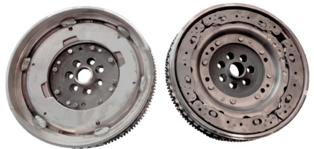
Bild 1: Optischer Vergleich von LuK-ZMS (links) und OE-ZMS (rechts)
