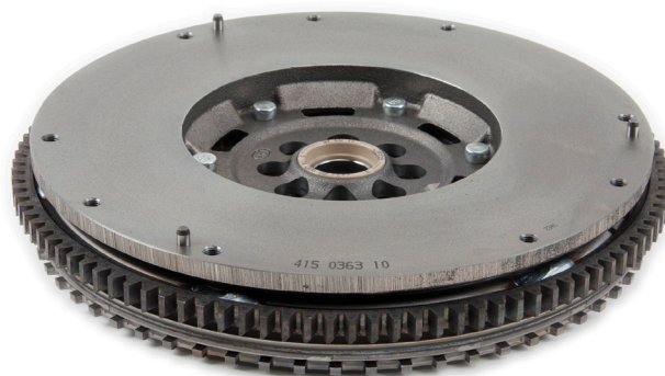
1. ábra: LuK DMF 415 0363 11
