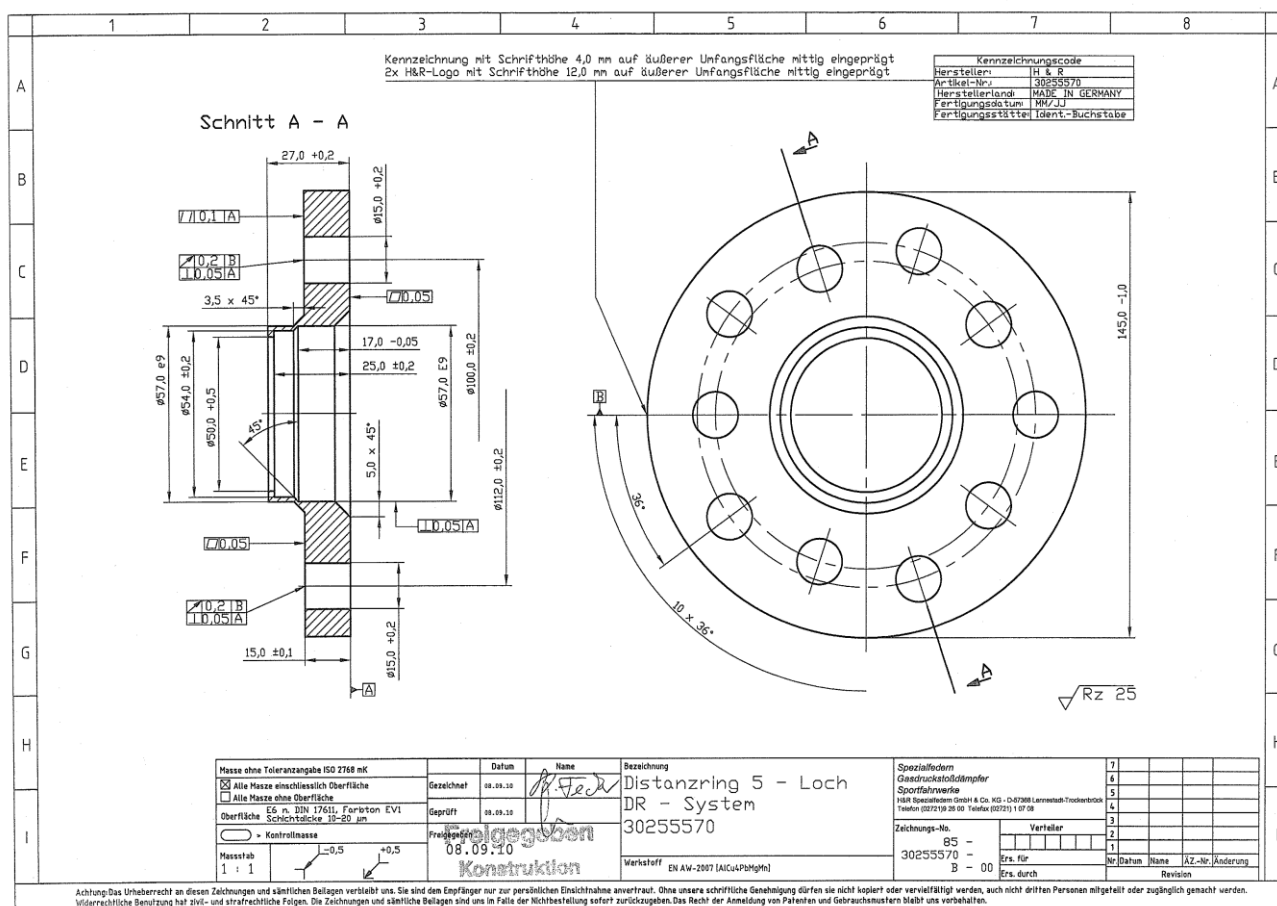
Zeichnung eines Distanzringes Nr. 30255570 vom 08.09.2010 (Beispiel)
