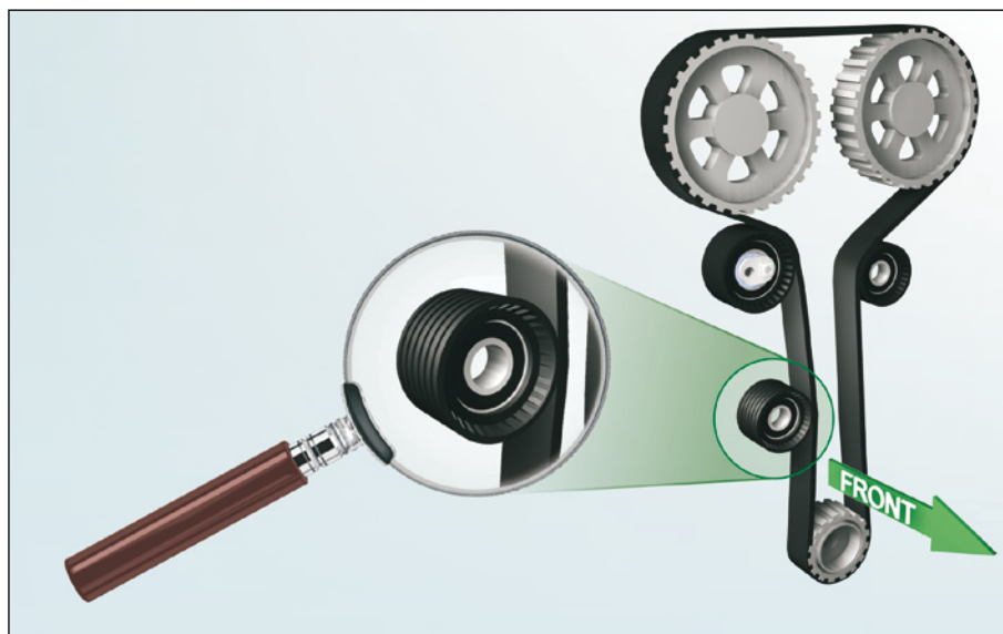
Bild 1: Riemenverlauf und Rollenpositionen im F4R-Motor
