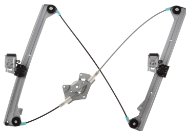
POWER WINDOW LEFT ALZACRISTALLI ELETTRICO SX
