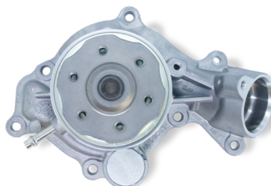
Bomba de agua 7.10942.38.0 con buje de seis orificios
