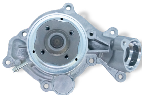
Bomba de agua 7.10942.21.0 con buje de cuatro orificios
