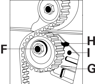
FIGURA 5 Allentare il bullone di bloccaggio F, agendo nel punto indicato, G, del tenditore automatico; portare l'indicatore mobile, H, nella posizione di massima tensione, e, dopo aver fatto coincidere il punto H con il Punto I, serrare il bullone di bloccaggio F.
