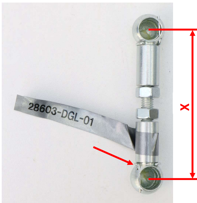
Abb. 2: Einstellmaß X HA
