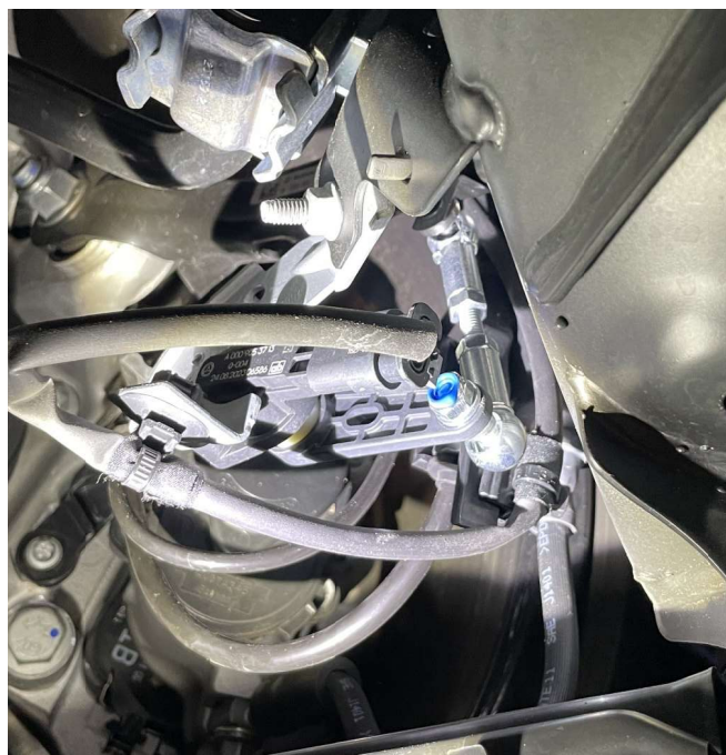
Abb. 1: Austausch der Niveauregelstangen HA (Abb. ähnlich) Fig. 1: Exchange of the level control rods RA (Fig. may vary)
