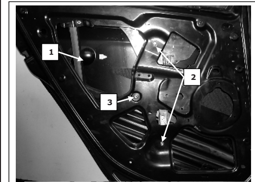
Porta lato sinistro, Portière arrière gauche, Left rear door, Puerta lado izquierdo, Hinten links Tür, Porta traseira esquerda, Sol arka kapi, νότρα οπίσθια αριστερή
