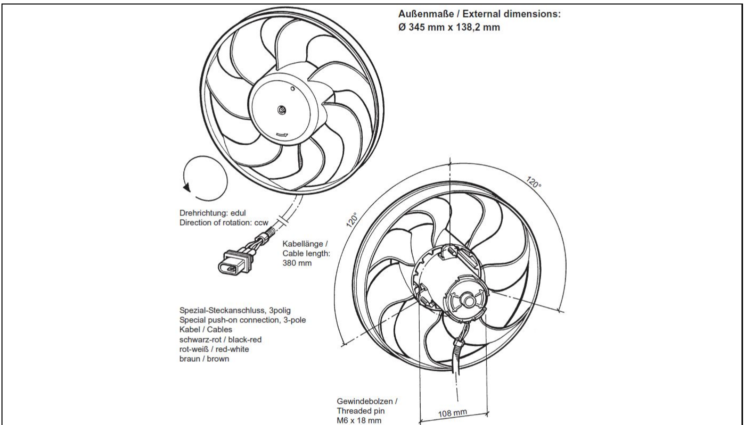
2 - Zeichnung / Drawing
