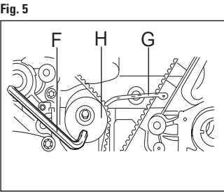
FIGURA 5 Girar el tensor de correa H en el sentido contrario a las agujas del reloj F y insertar la herramienta para inmovilización del tensor de correa G.
