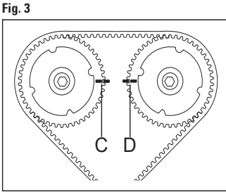
FIGURA 1 Verificar la correcta alineación de los arboles de leva A. FIGURA 2 Verificar el posicionamiento correcto la herramienta de inmovilización de árbol de levas B. FIGURA 3 Verificar el posicionamiento correcto de las marcas de fase C y D. FIGURA 4 Insertar la herramienta especial de inmovilización de árbol de levas E.
