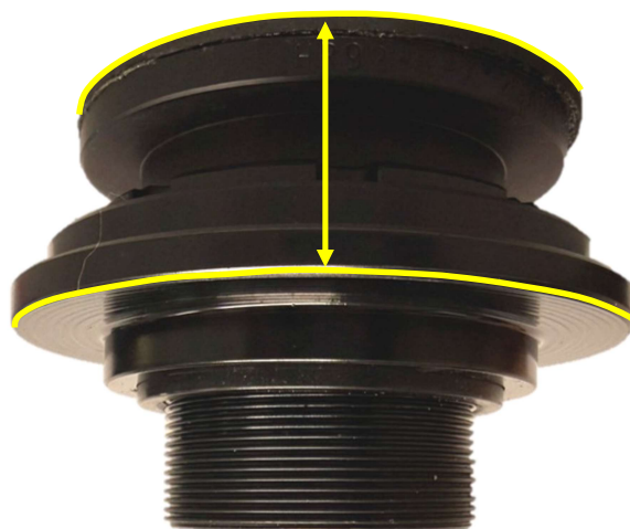
Abb. 6: Einstellmaß HA (Abbildung ähnlich)
