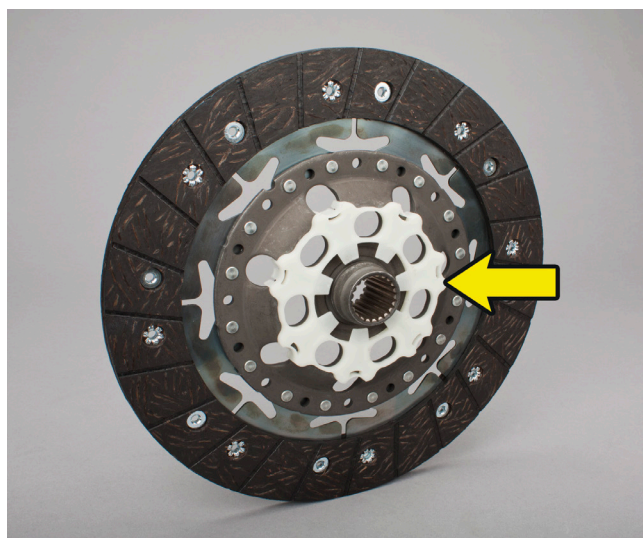
1. ábra: LuK kuplungtárcsa műanyag gyűrűvel
