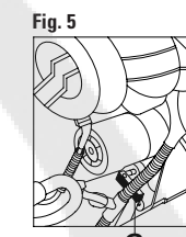
FIGURA 4 Verificar la correcta alineación de las marcas de puesta en fase E y F. FIGURA 5 Insertar la herramienta de inmovilización del volante motor G.
