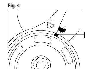
FIGURA 3 Controllare il corretto allineamento delle tacche di fase H. FIGURA 4 Controllare il corretto allineamento delle tacche di fase I.
