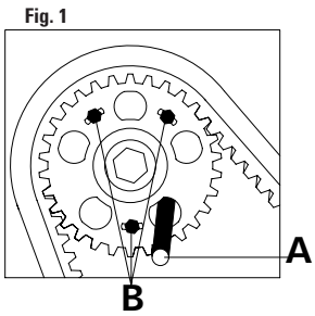
FIGURA 1 Insertar la herramienta especial de inmovilización de árbol de levas A. Los tornillos B, no deben estar situados en la extremidad de las acanaladuras.
