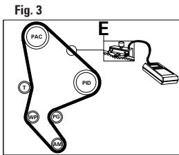
FIGURA 2 Allentare il bullone di bloccaggio C e ruotare il tendicinghia in senso antiorario tramite l'attrezzo di tensionamento inserito in D fino alla corretta misura di tensione; serrare quindi il bullone di bloccaggio C. FIGURA 3 Inserire l'apposito attrezzo di misura del tensionamento E, nel punto indicato, ed agire sul tendicinghia fino al valore di 51±3 unità SEEM.
