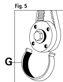
FIGURA 4 Inserire l'apposito attrezzo di bloccaggio del volano F. FIGURA 5 Inserire l'apposito attrezzo di bloccaggio della cinghia di distribuzione G.
