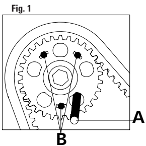
FIGURA 1 Inserire l'apposito attrezzo di bloccaggio dell'albero a camme A. I bulloni B non devono trovarsi all'estremità delle scanalature.
