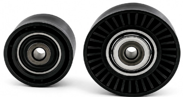
Bild 2: Umlenkrollen mit neuem Dichtungskonzept (ohne Abdeckkappe)
