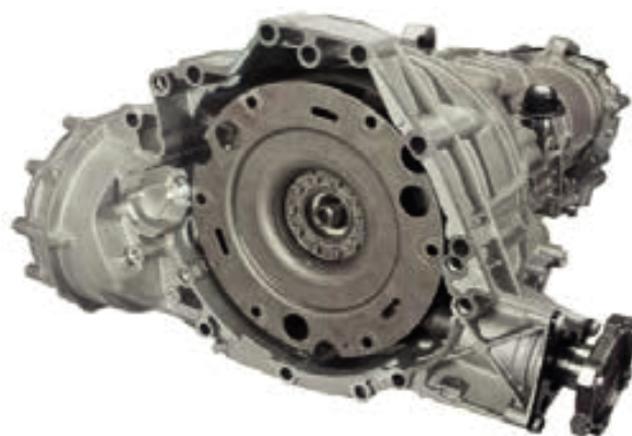
Foto 1: Skrzynia biegów z osadzonym modulem sprzęgła
