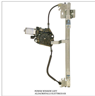
POWER WINDOW LEFT ALZACRISTALLI ELETTRICI ESX
