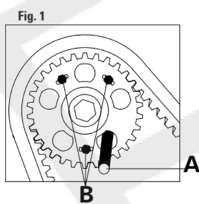
FIGURA 1 Inserire l'apposito attrezzo di bloccaggio dell'albero a camme A. I bulloni B non devono trovarsi all'estremità delle scanalature.
