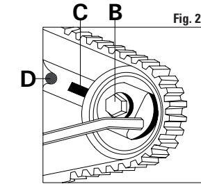
FIGURA 2 Aflojar el tornillo de fijación B, girar el tensor de correa en sentido contrario a las agujas del reloj, alinear el indicador C en el centro de la zona de control D. Luego proceda apretar el tornillo de fijación B.
