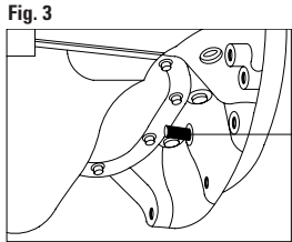
FIGURA 3 Inserire l'apposito attrezzo di bloccaggio del volano E. FIGURA 4 Ruotare l'albero motore fino ad allineare il foro per la messa in fase del motore ed installare, quindi, l'apposito attrezzo di bloccaggio F.
