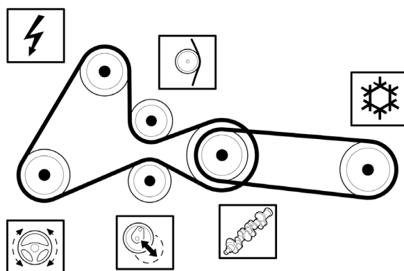
2. ábra: Ékszíjhajtás a 0113090 motorszámtól elasztikus hosszbordás ékszíjjal
