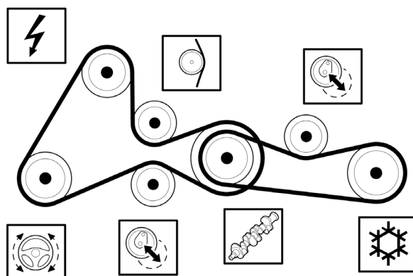
1. ábra: Ékszíjhajtás a 0113089 motorszámtól feszítőgörgővel
