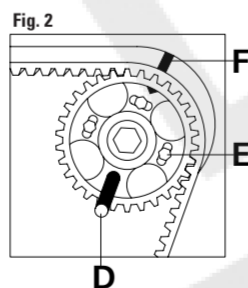
FIGURA 1 Inserire l'apposito attrezzo di bloccaggio dell'albero a camme A. Allineare i punti di fase B. I bulloni C non devono trovarsi all'estremità delle scanalature. FIGURA 2 Inserire l'apposito attrezzo di bloccaggio dell'albero a camme D. Allineare i punti di fase E. I bulloni F non devono trovarsi all'estremità delle scanalature.
