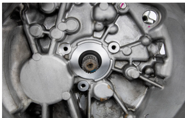
1. ábra: A központi kinyomó felfekvő felülete a sebességváltó házában
