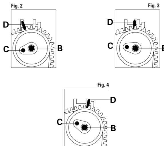
FIGURA 2 Allentare il bullone di bloccaggio B e ruotare in senso orario il tendicinghia sull'eccentrico di registro C, ed allineare l'indicatore D nella zona di controllo. Serrare, quindi, il dado di bloccaggio B. Tensione alla temperatura di -20° C FIGURA 3 Allentare il bullone di bloccaggio B; ruotare in senso orario il tendicinghia sull'eccentrico di registro C, ed allineare l'indicatore D nella zona di controllo; serrare quindi il dado di bloccaggio B. Tensione alla temperatura di 20° C. FIGURA 4 Allentare il bullone di bloccaggio B; ruotare in senso orario il tendicinghia sull'eccentrico di registro C, ed allineare l'indicatore D nella zona di controllo; serrare, quindi, il dado di bloccaggio B. Tensione alla temperatura di 50° C.
